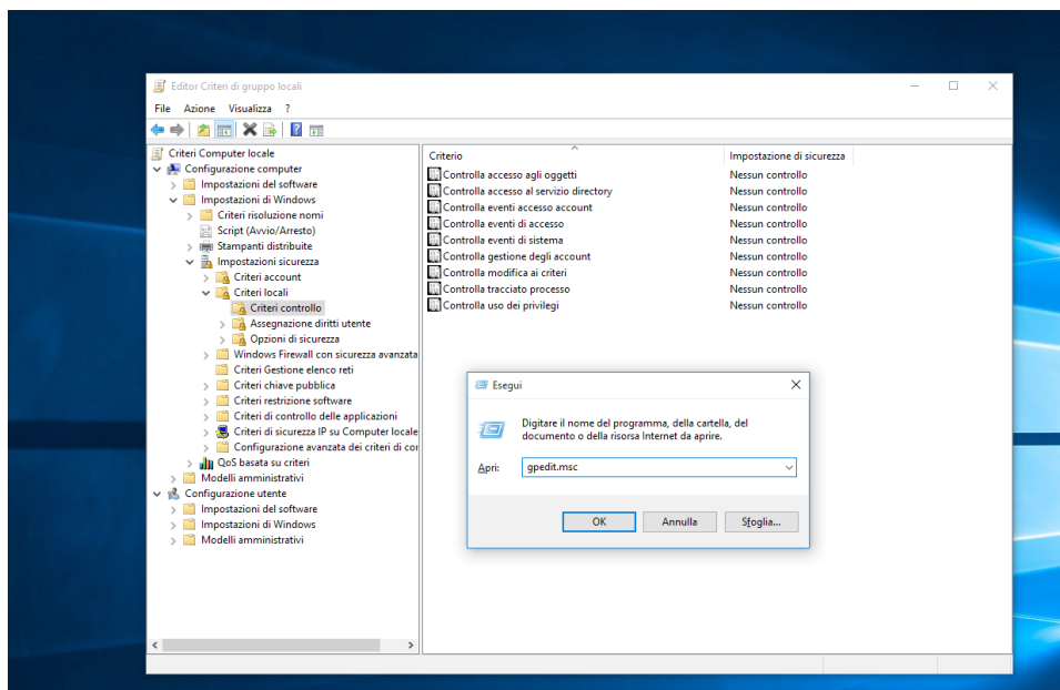
Figura 3 – Apertura dell'Editor Criteri di gruppo locali (gpedit.msc) e visualizzazione dei Criteri di controllo.
