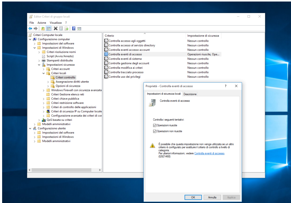
Figura 4 – Abilitazione del controllo per il criterio "Controlla eventi di accesso" (operazioni riuscite e non riuscite).
